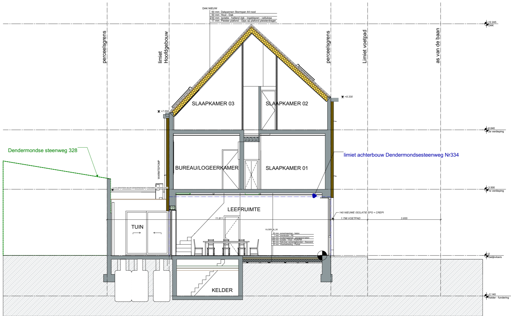
Maateenheid: Millimeter Snede A-A NT Schaal : 1:100
