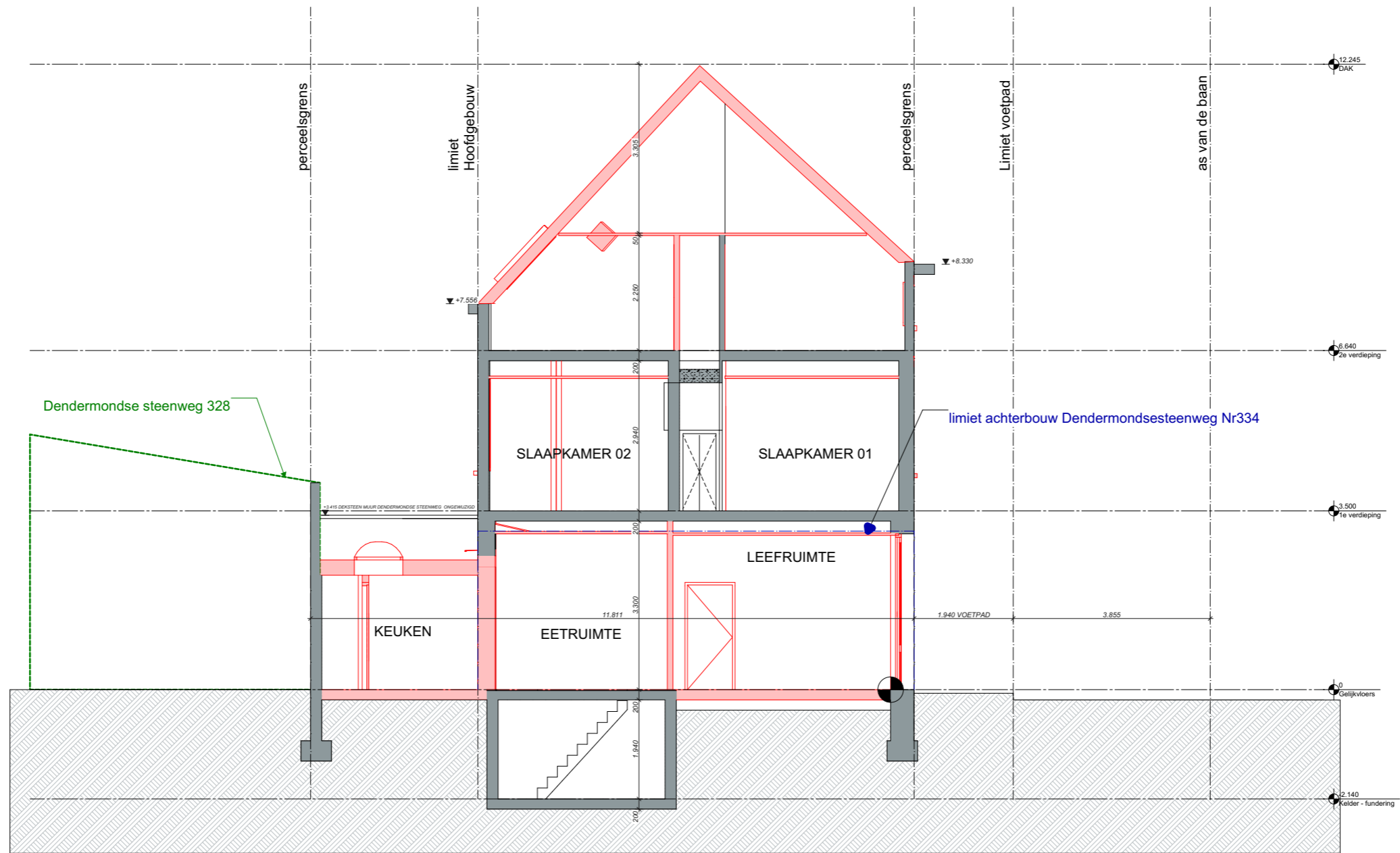
Maateenheid: Millimeter Terreinprofiel 01 BT Schaal : 1:100
