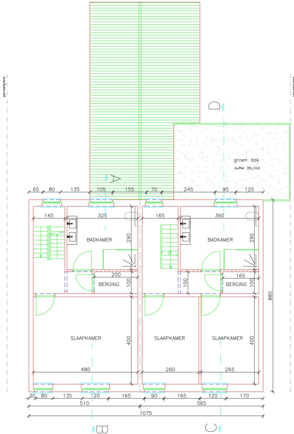
BA woning-P-N-2-verdieping 1
