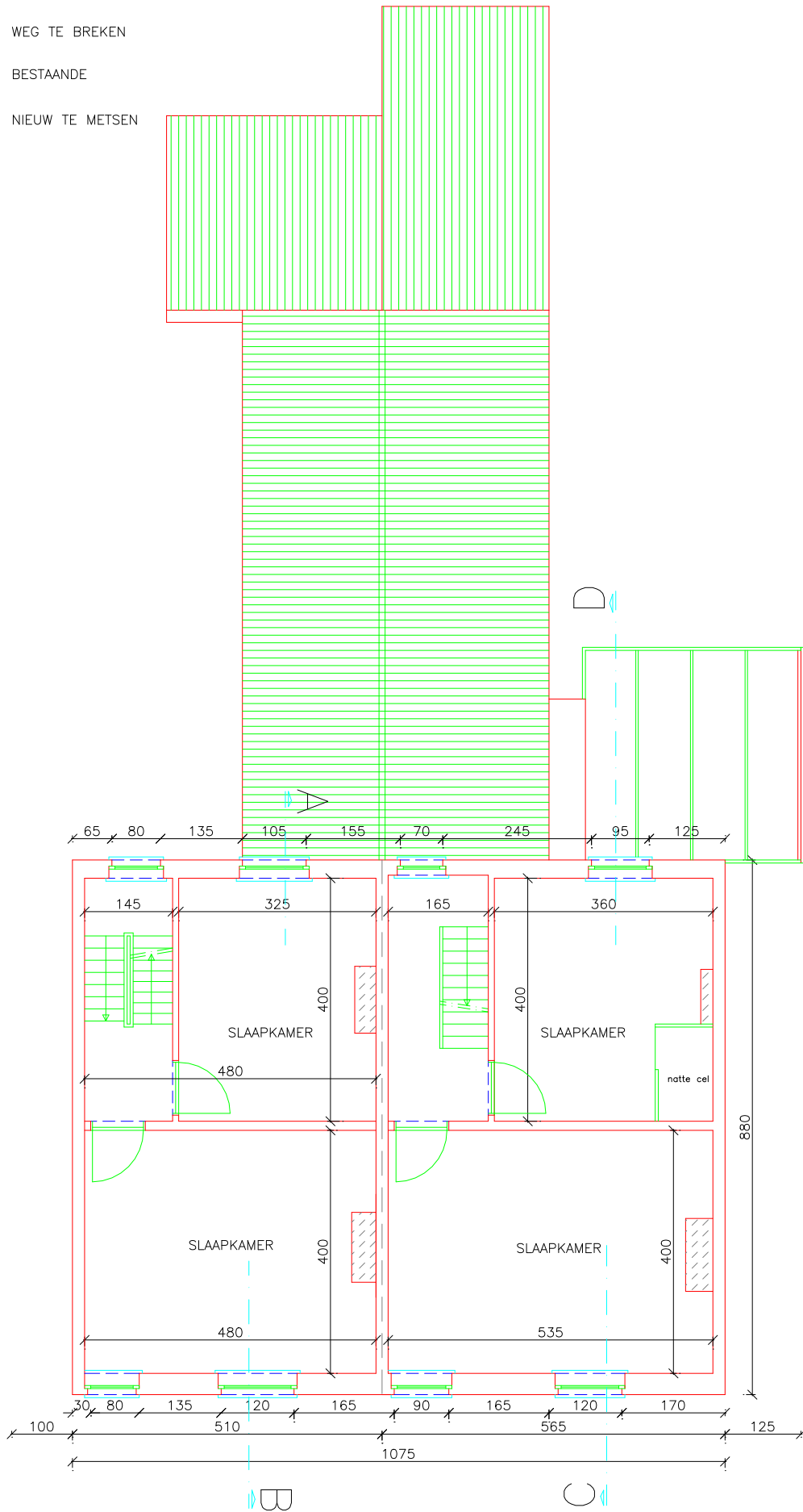
BA woning-P-B-2-verdieping 1
