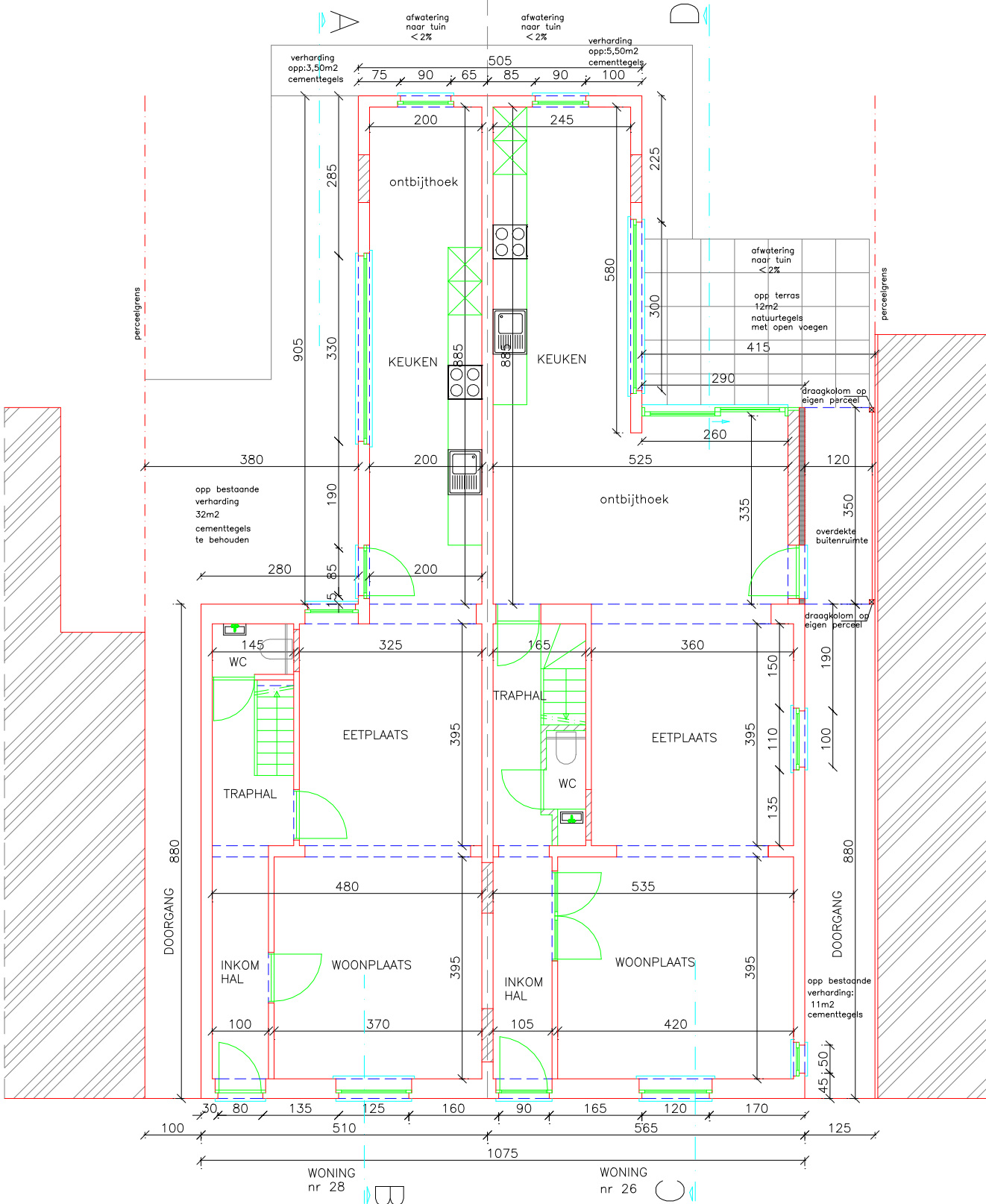
BA woning-P-N-1-gelijkvloers
