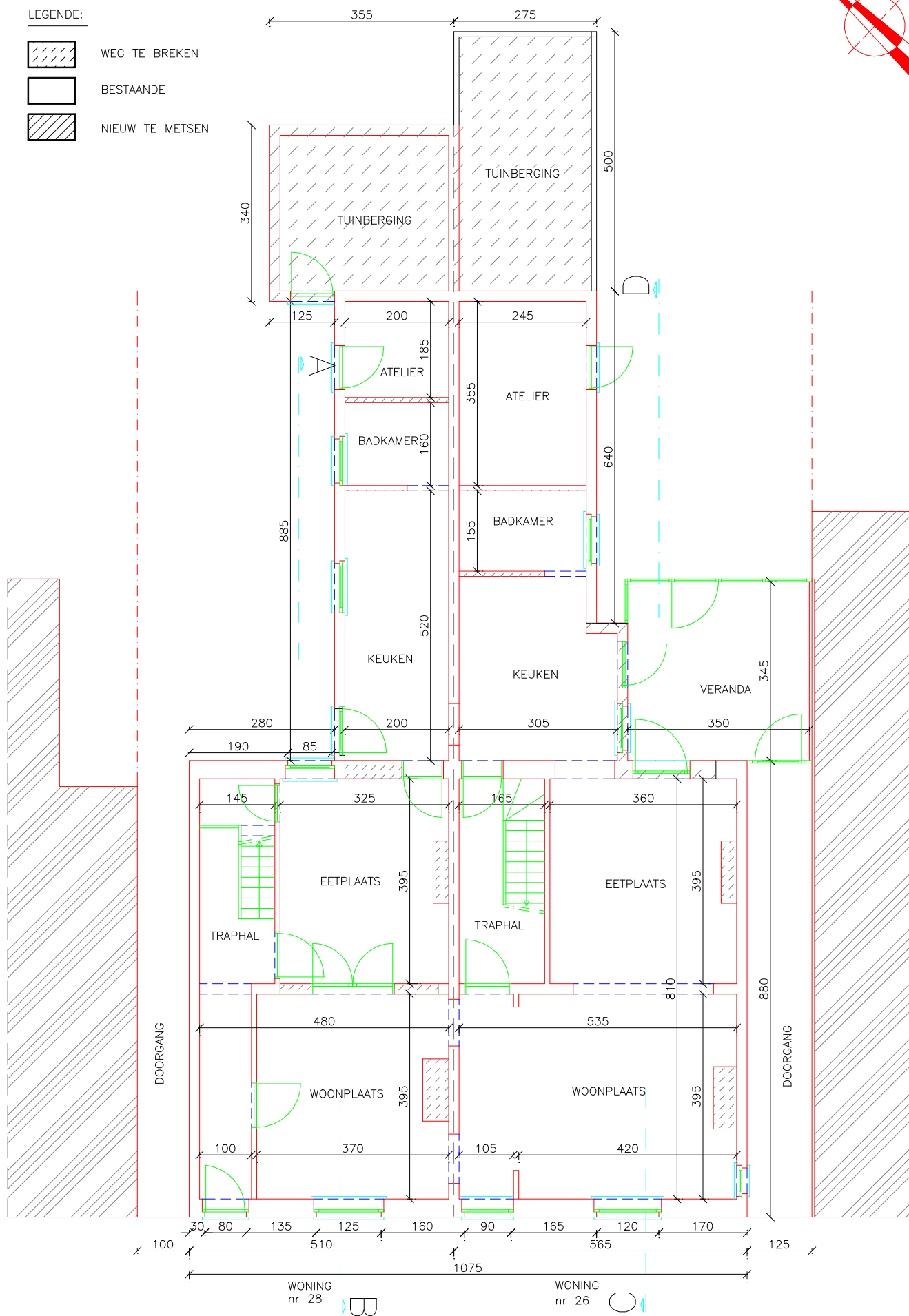
BA woning-P-B-1-gelijkvloers
