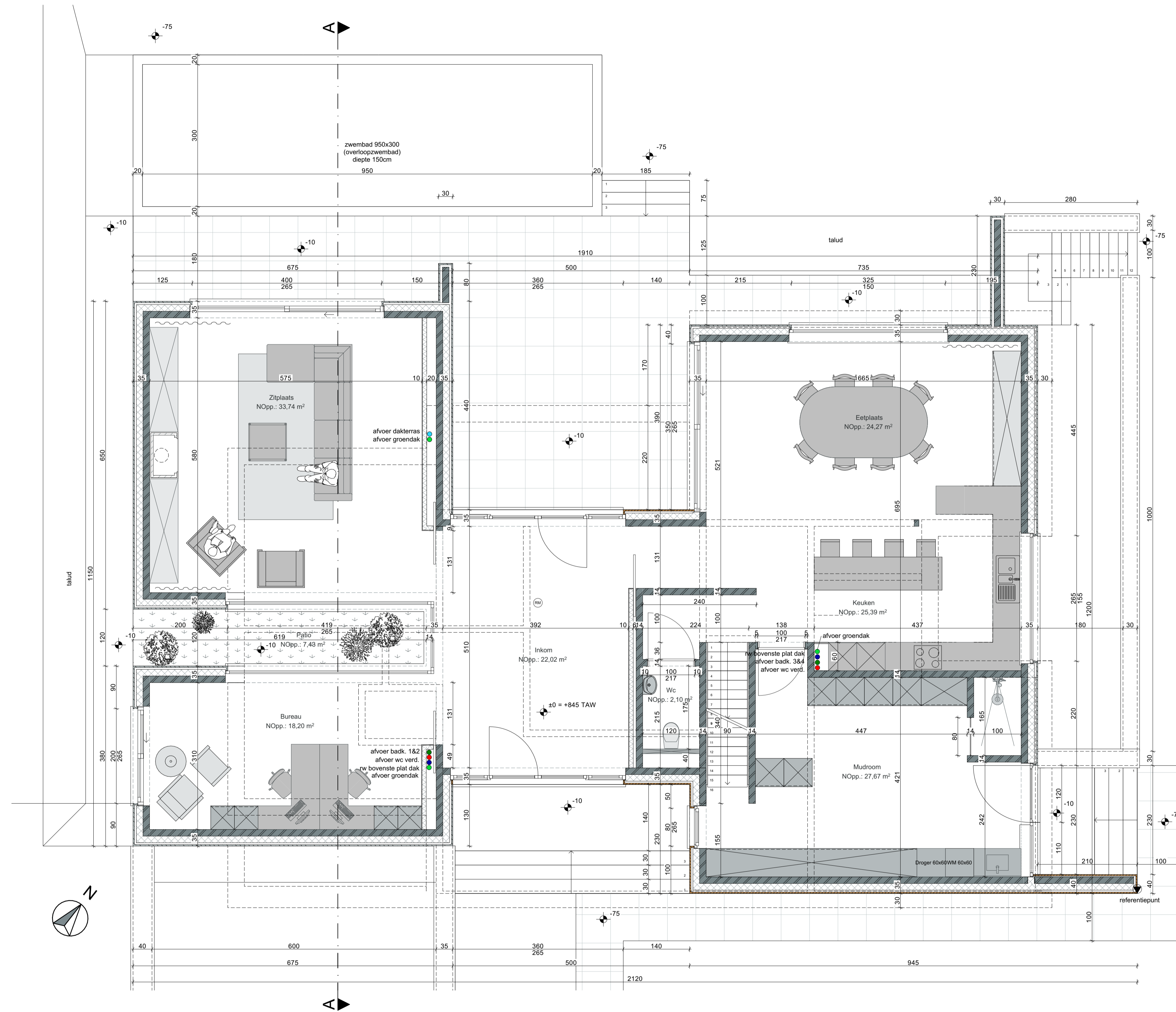
GRONDPLAN GELIJKVLOERS
