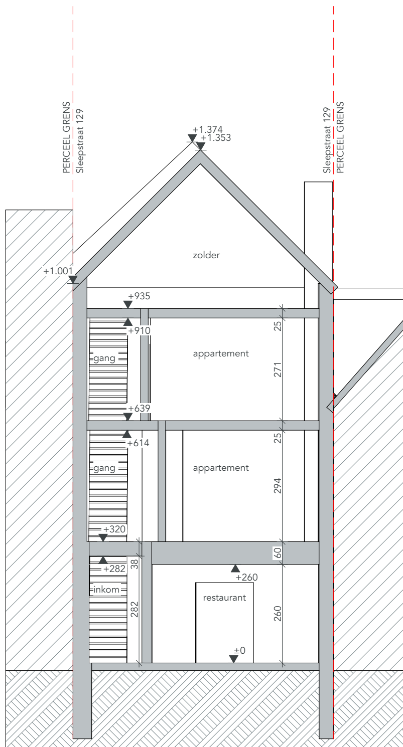
VT Doorsnede A-A
