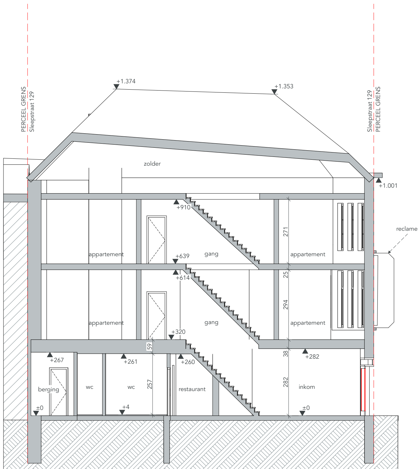
BT Doorsnede B-B
