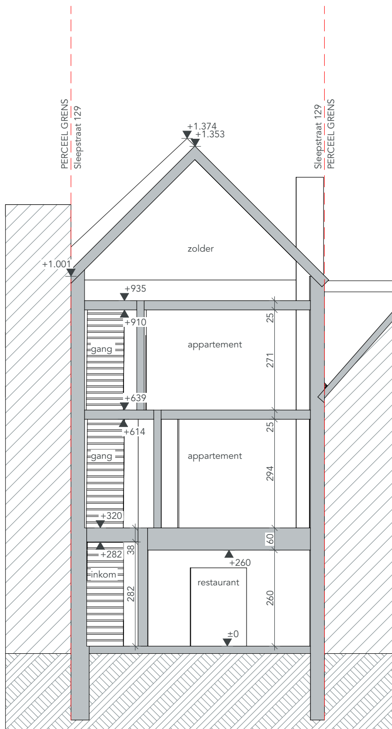
BT Doorsnede A-A
