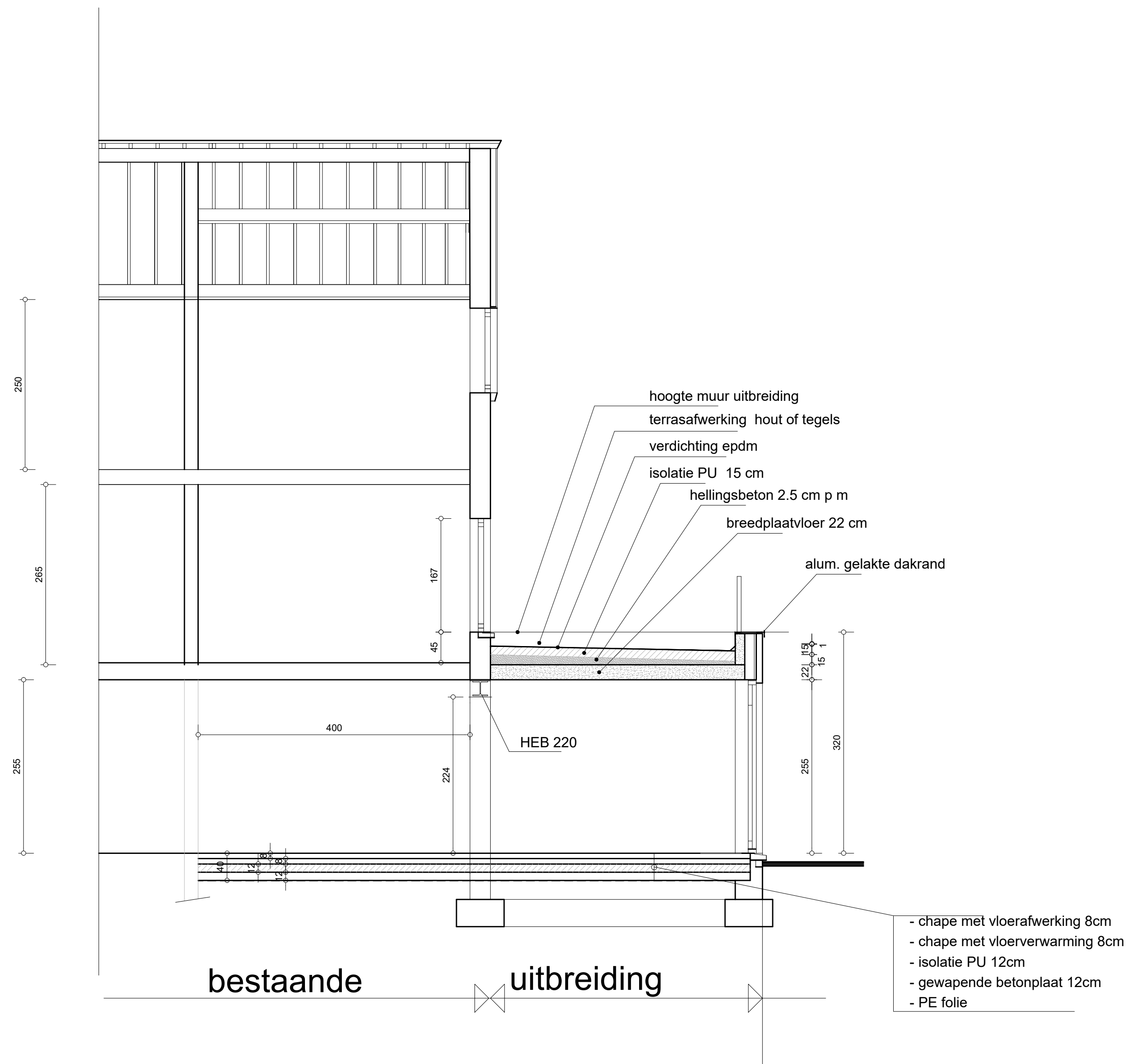
STRUKTUUR DOORSNEDE C-D NIEUWE TOESTAND
