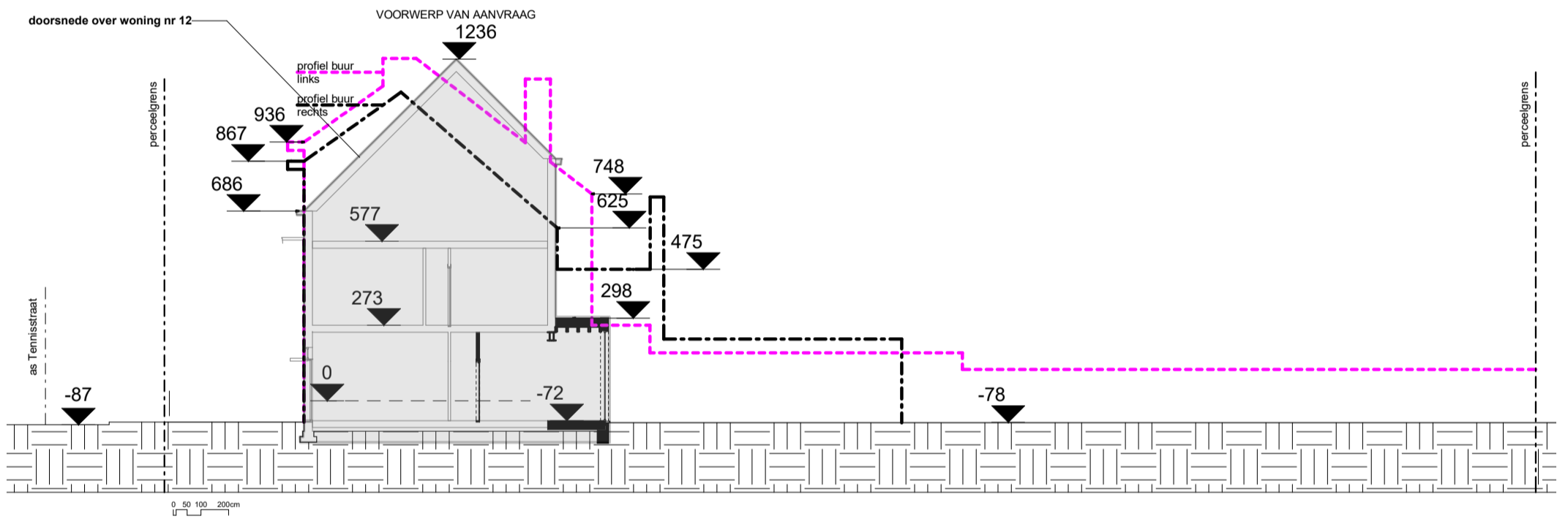
Terreinprofiel (zie: Terreindoorsnede 1)
