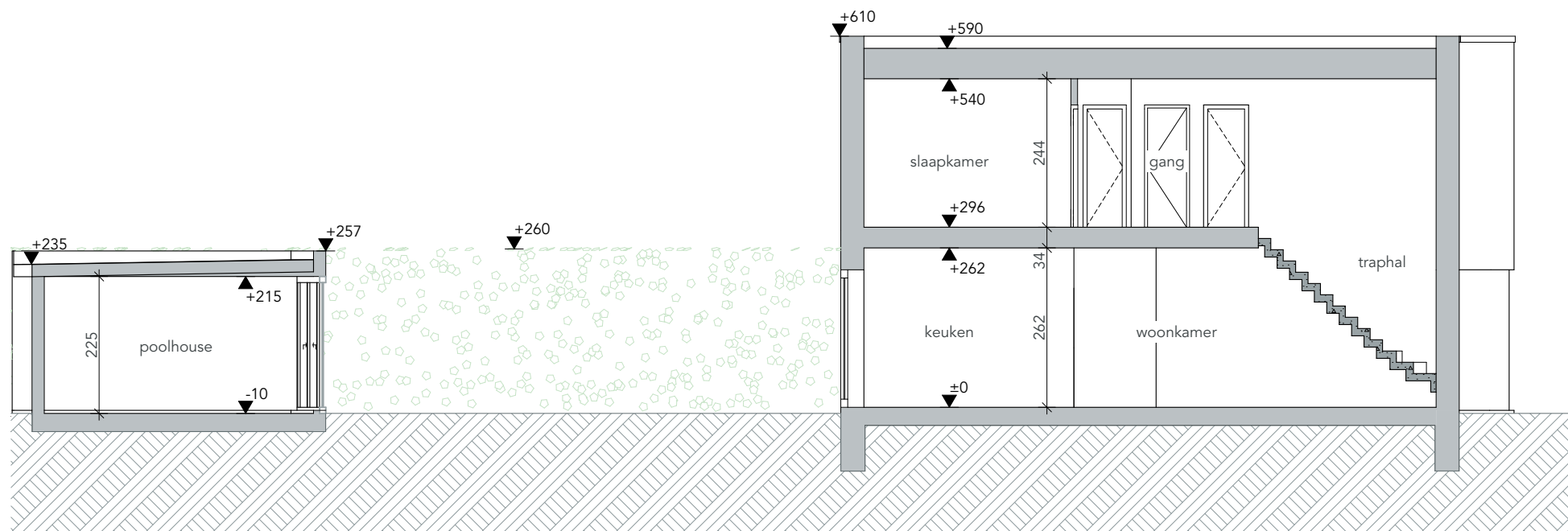
NT Doorsnede B-B
