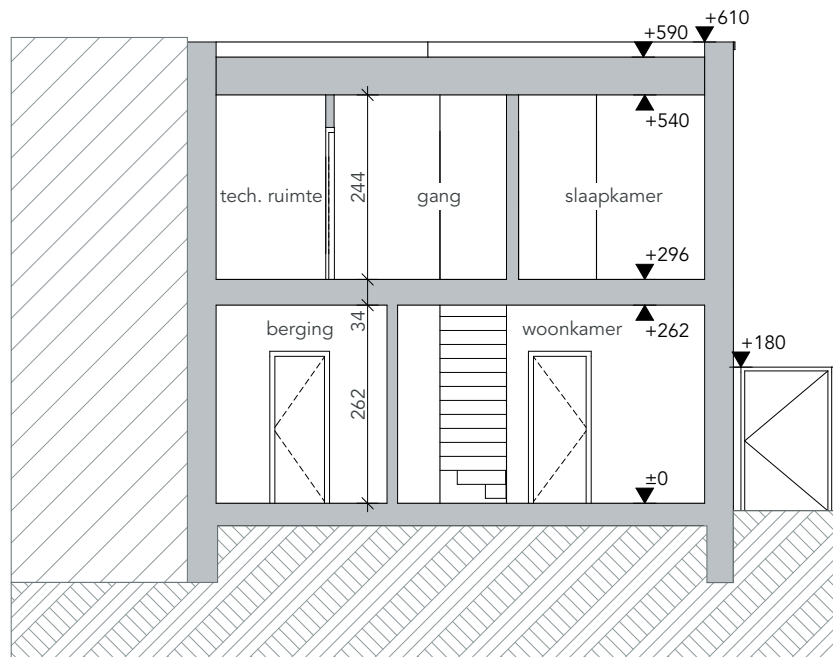
NT Doorsnede A-A
