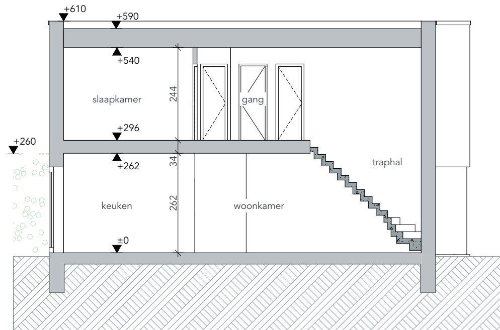
0 1 2 3 4 VT Doorsnede B-B
