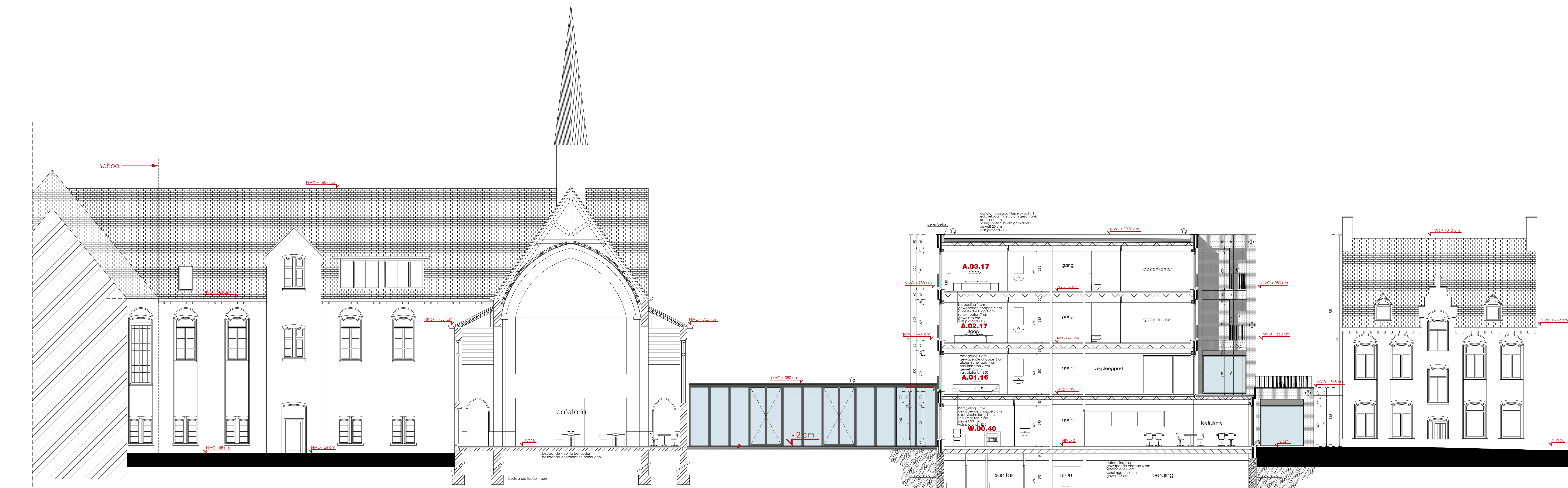
doorsnede G-G gevel NOORD-WEST - binnentuin
