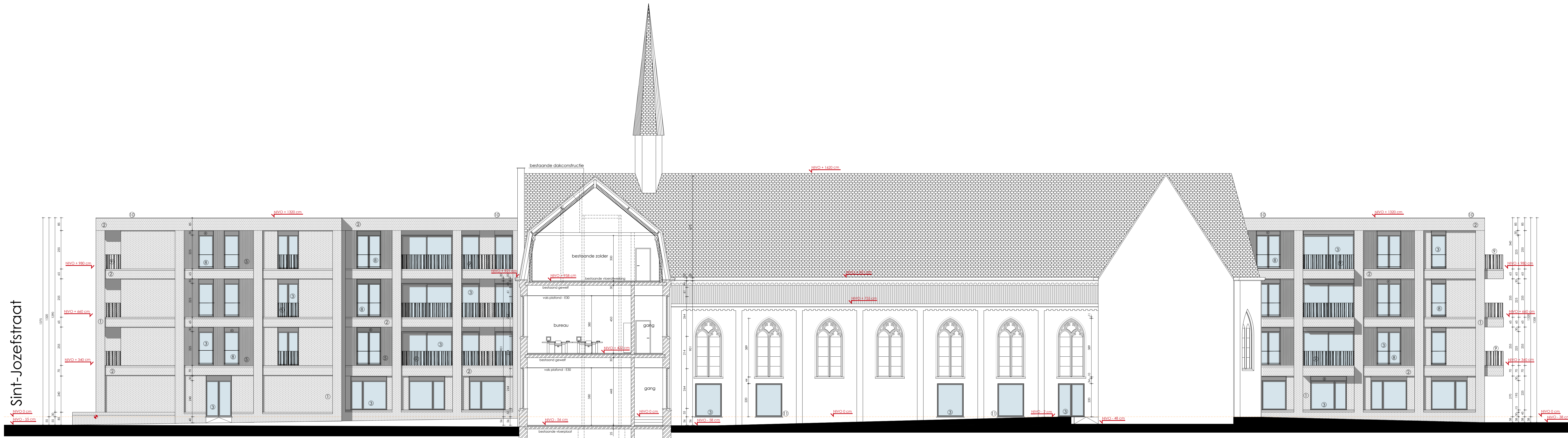
doorsnede J-J gevel NOORD-OOST - inkompleintje
