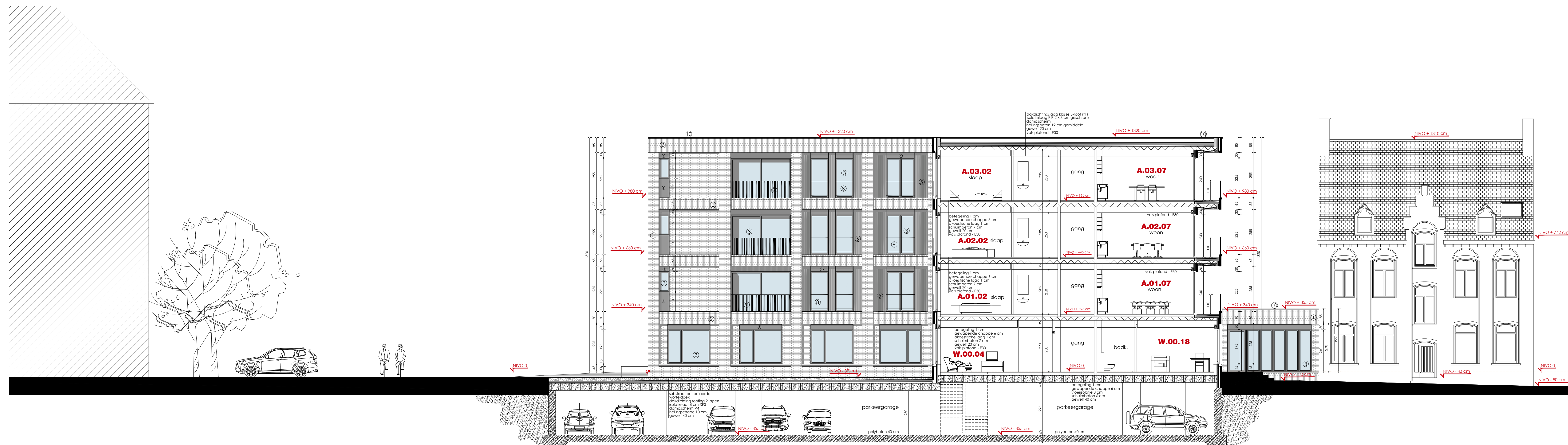
doorsnede H-H gevel NOORD-WEST - inkompleintje
