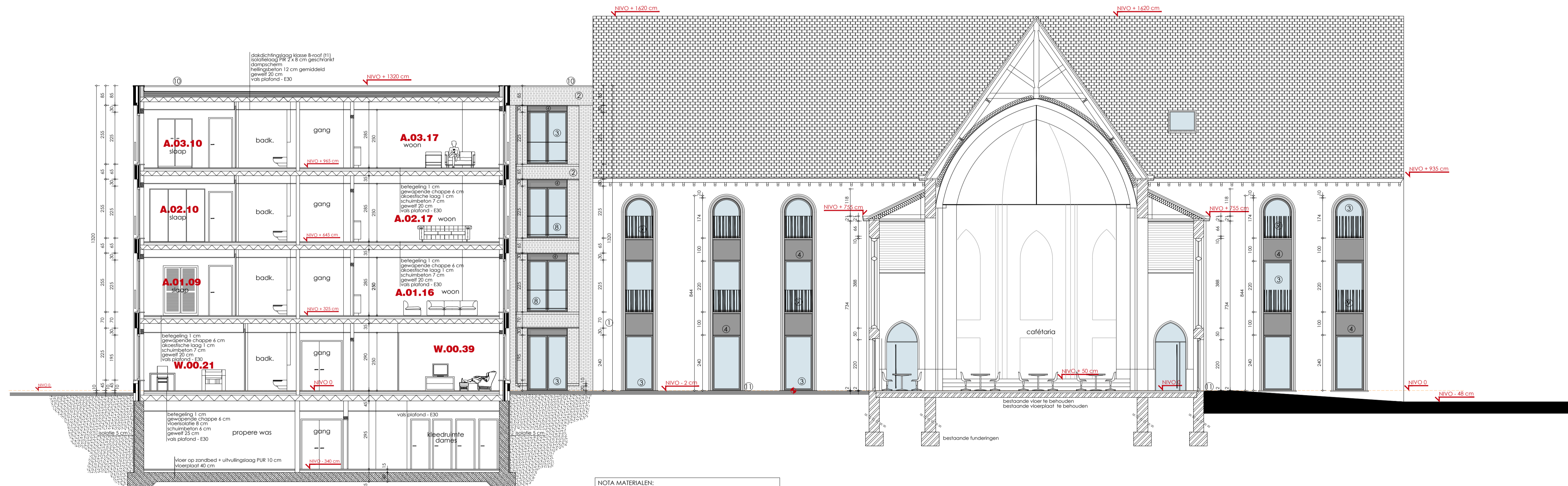
doorsnede C-C gevel ZUID-OOST - binnentuin
