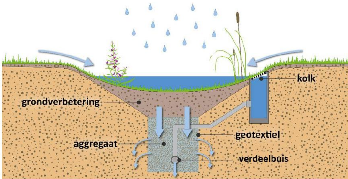
Figuur 20: opbouw van een wadi (blaugroenvlaanderen)
