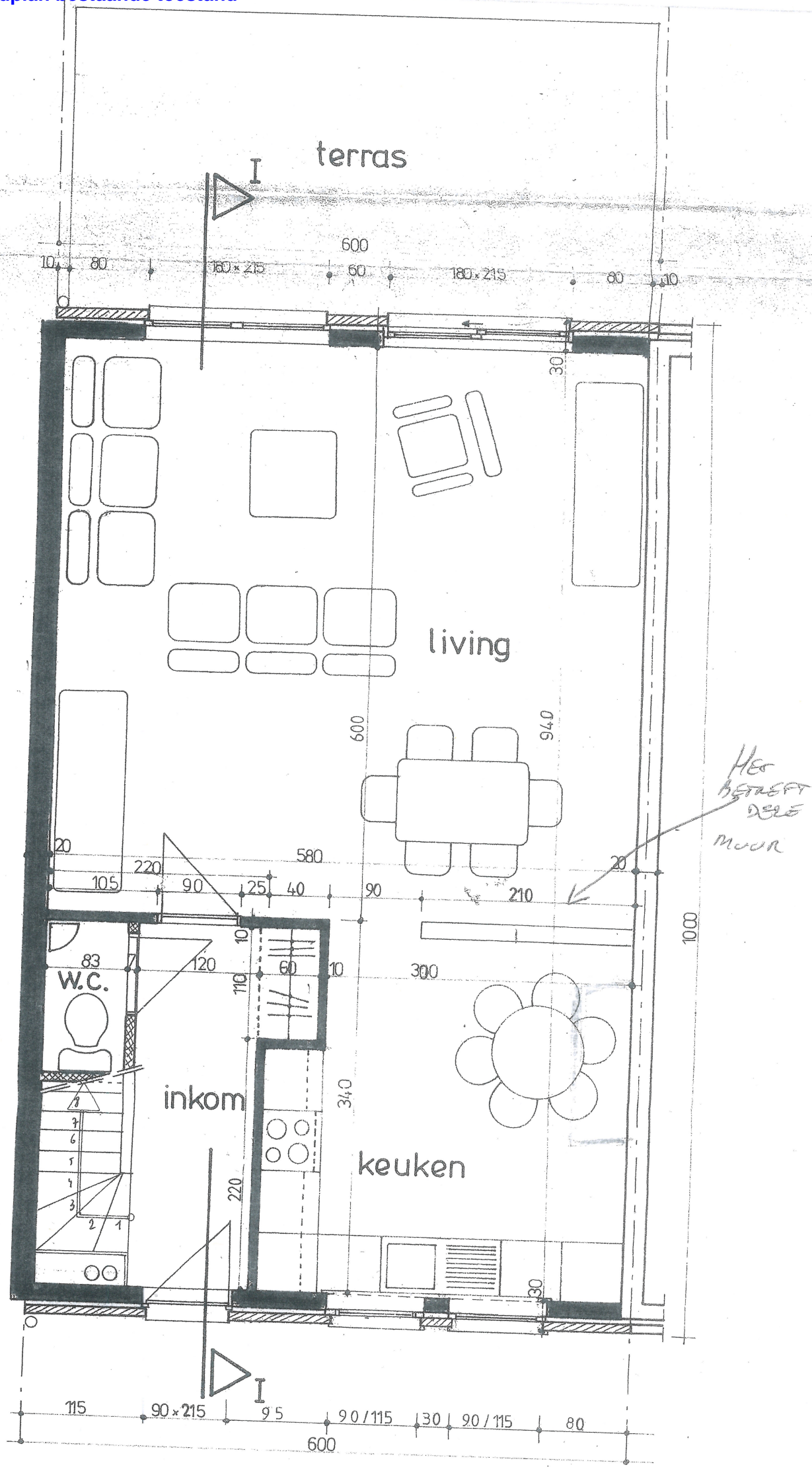
GRONDPLAN BT 1/50.
