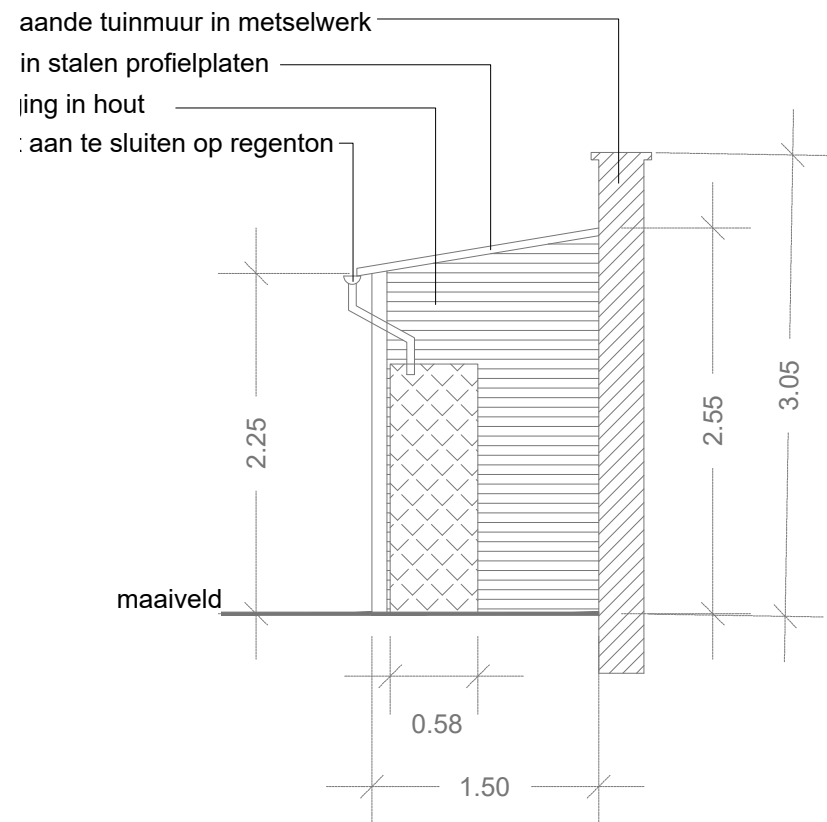
ZIJAANZICHT LINKS
