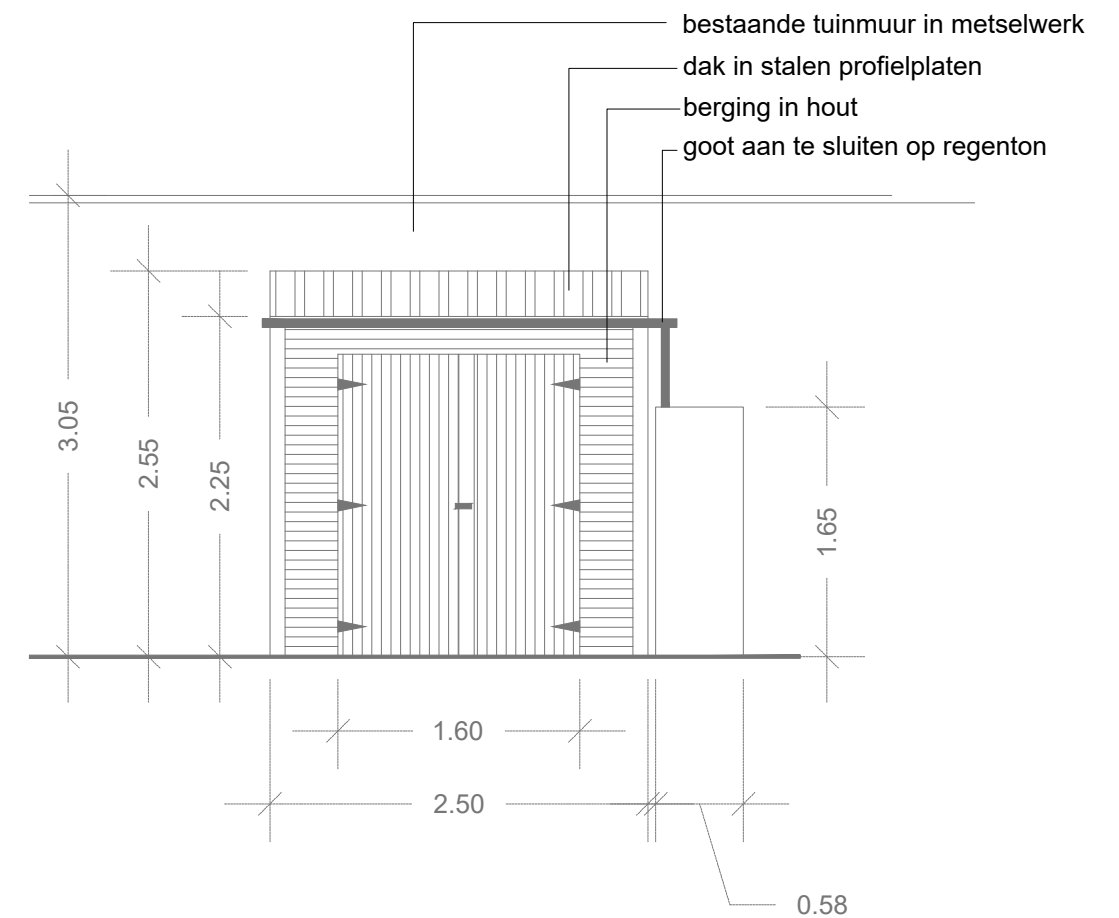
VOORAANZICHT
