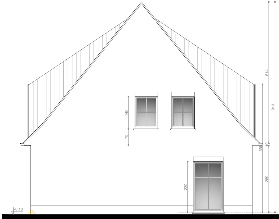
RECHTER ZIJGEVEL
