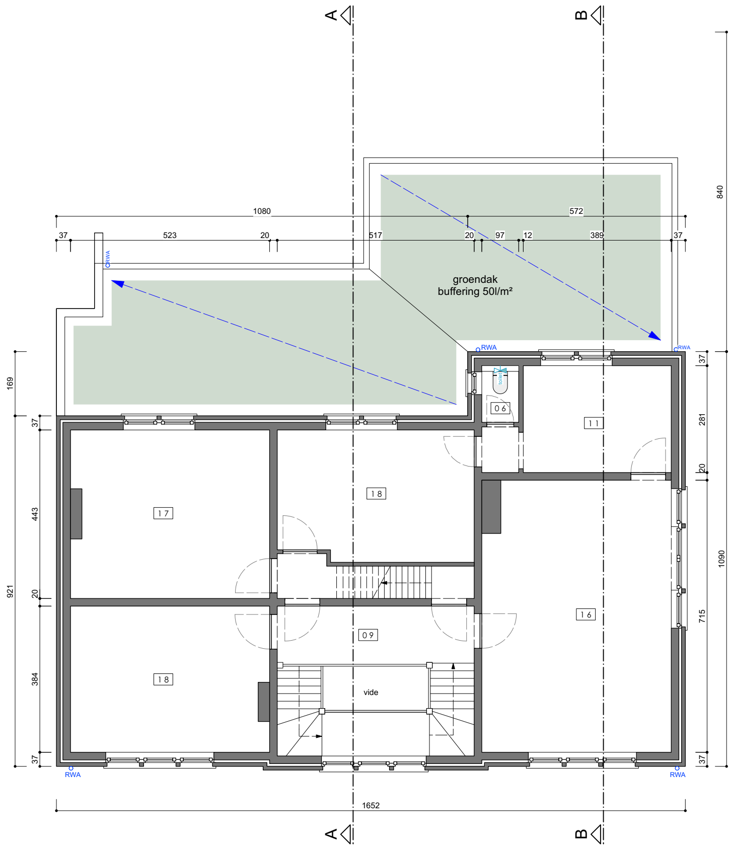
VERDIEPING +1 nieuwe toestand schaal 1/100
