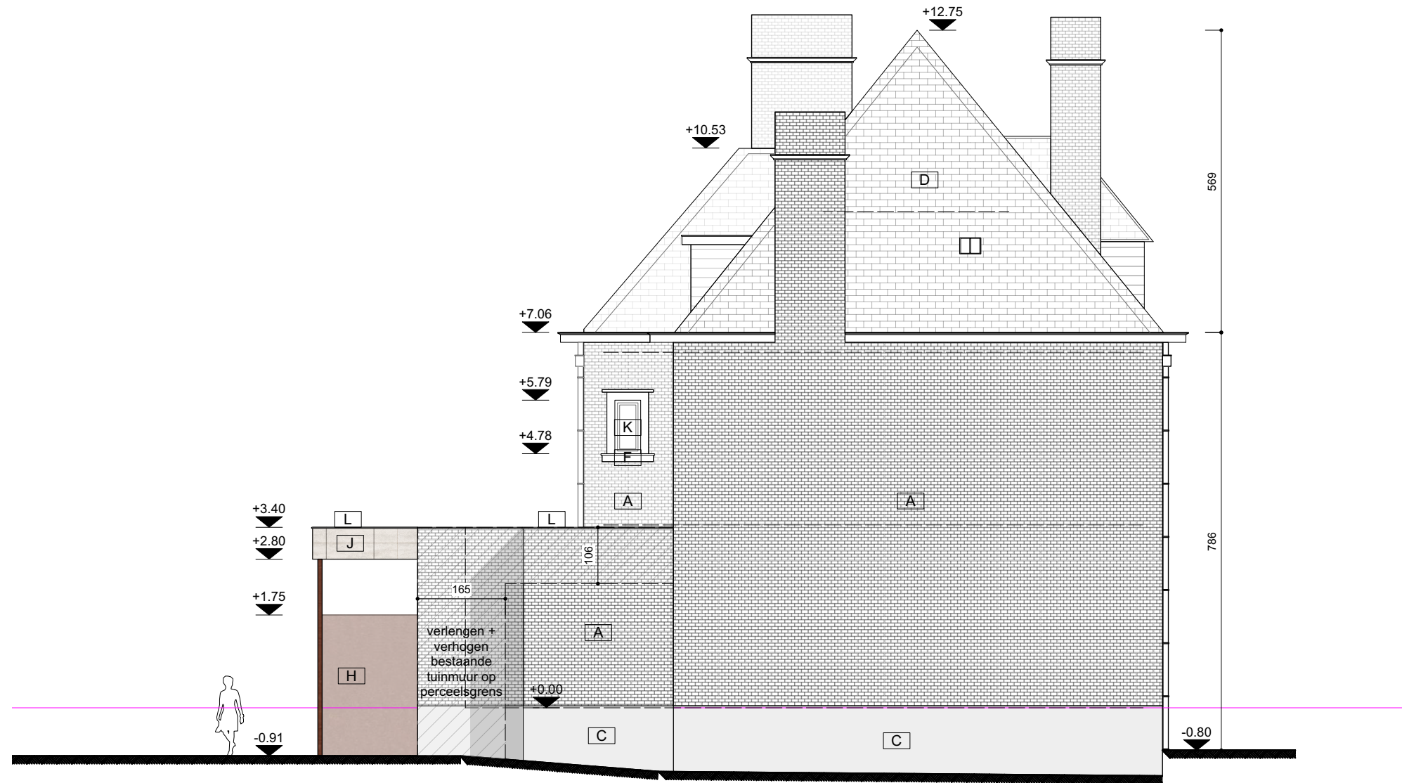
ZIJAANZICHT LINKS nieuwe toestand schaal 1/100
