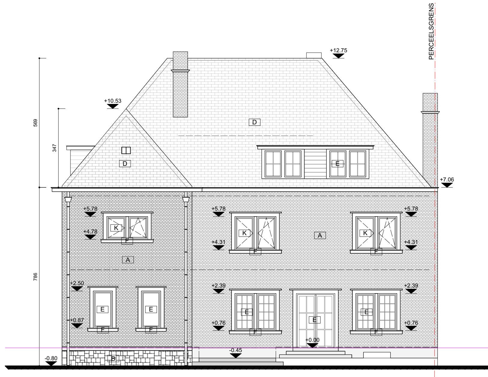
ACHTERAANZICHT bestaande toestand schaal 1/100
