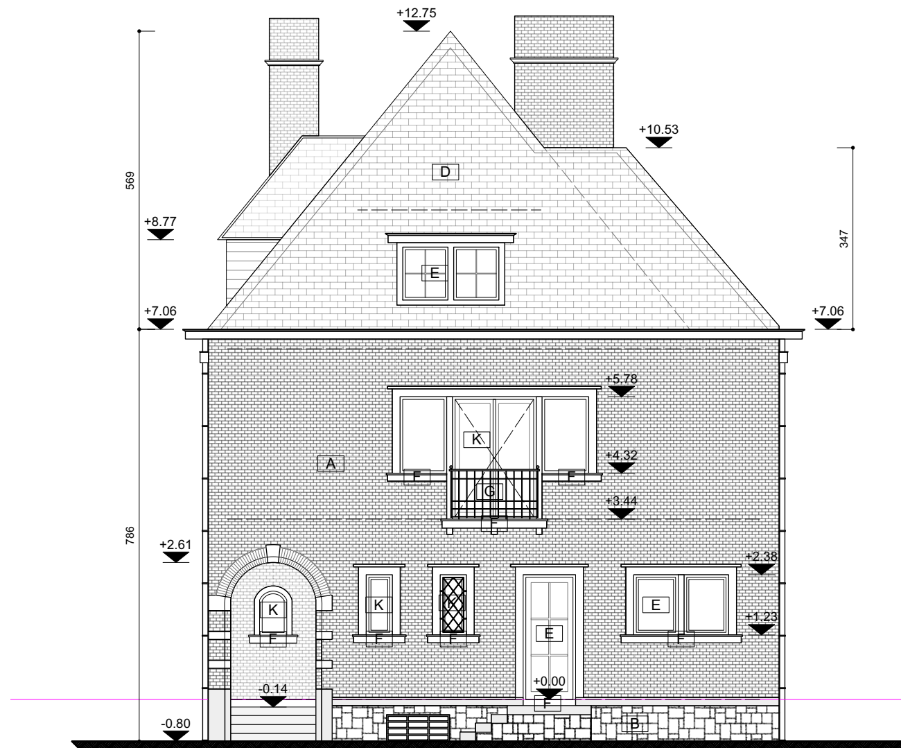
ZIJAANZICHT RECHTS bestaande toestand schaal 1/100
