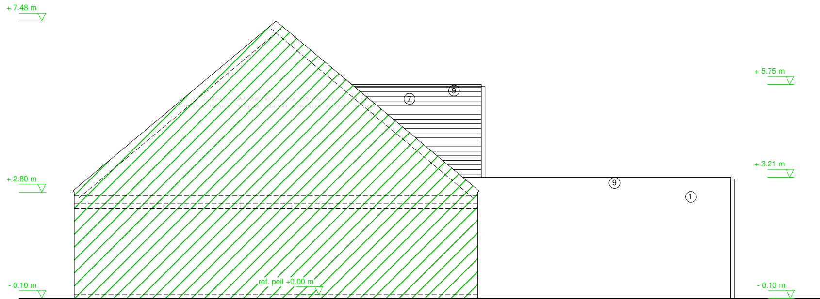
ZIJGEVEL RECHTS nieuwe toestand
