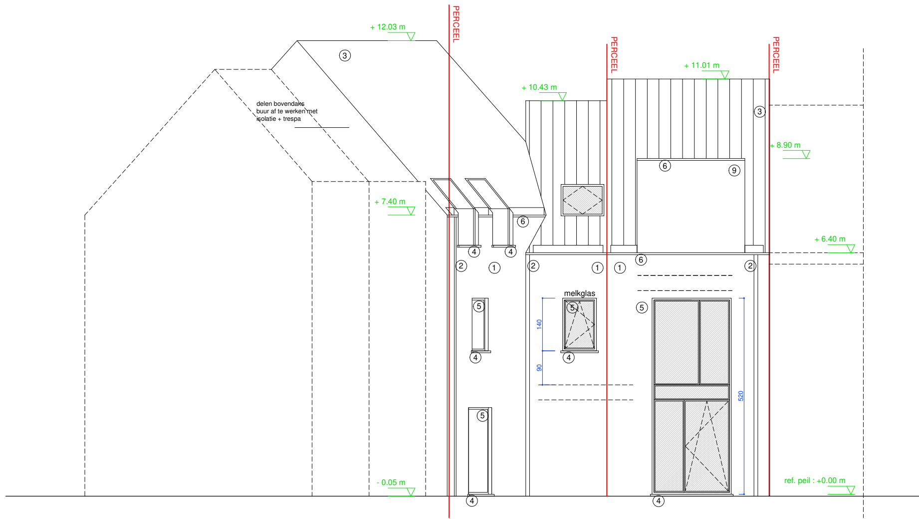
ACHTERGEVEL EEKHOUTDRIESSTRAAT nieuwe toestand
