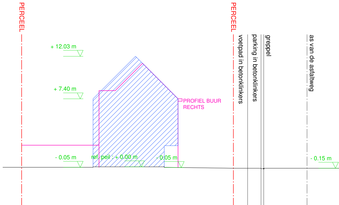
TERREINPROFIEL 2 nieuwe toestand schaal 1/200
