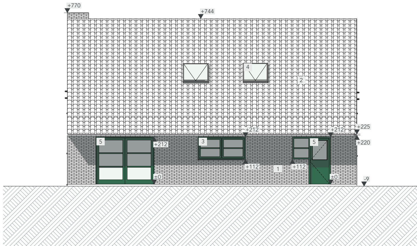
0 1 2 3 4 BT Achtergevel
