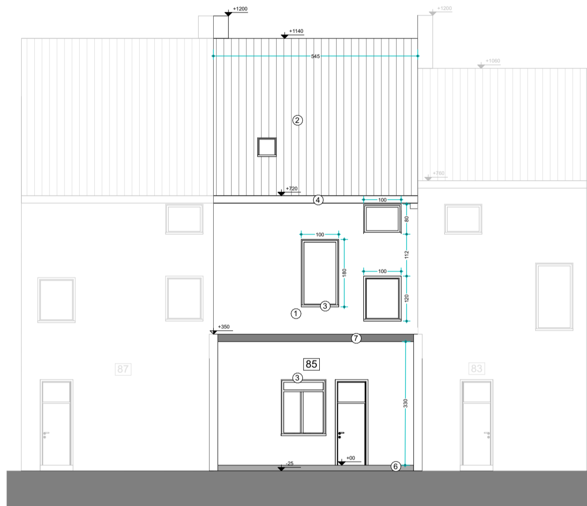
BESTAANDE ACHTERGEVEL
