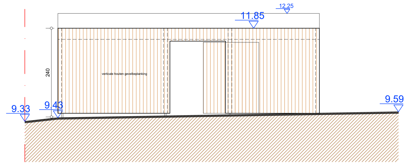
zijgevel fietsenberging
