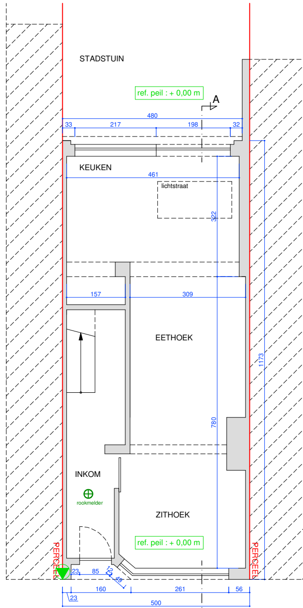
GRONDPLAN bestaande toestand ongewijzigd
