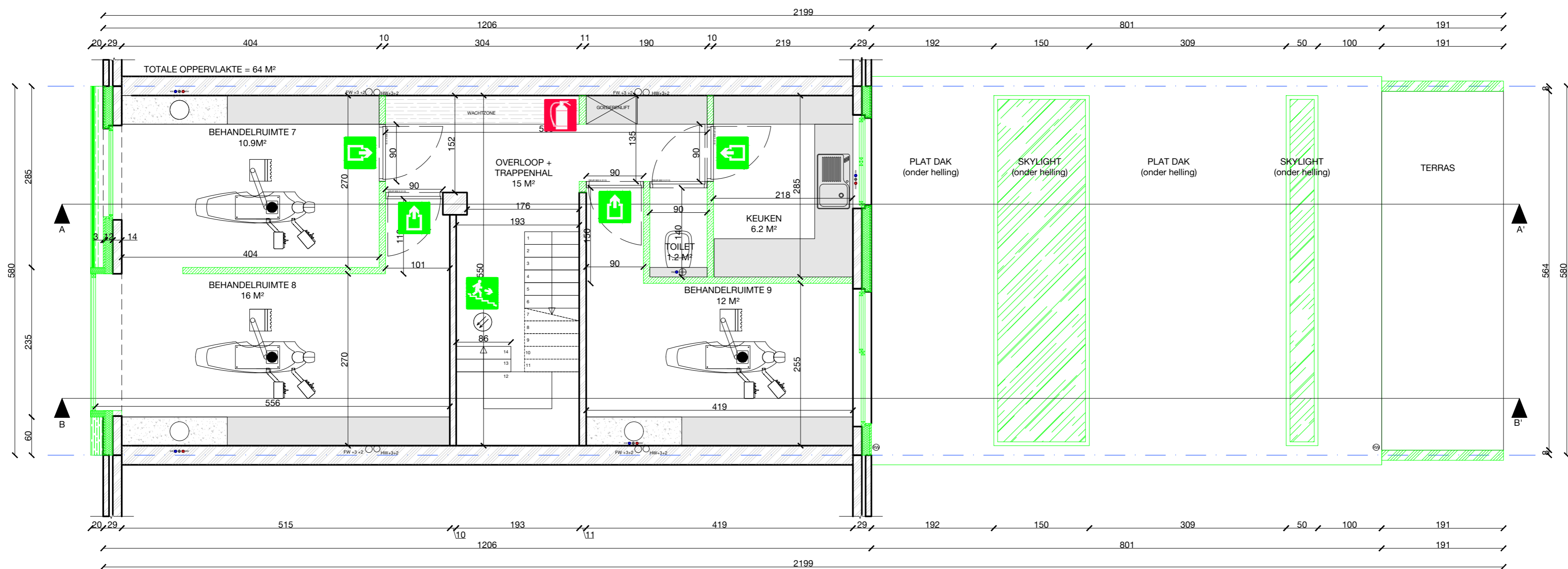
GRONDPLAN VERDIEPING +2- VERGUNDE SITUATIE (reeds verleend) 1:50
