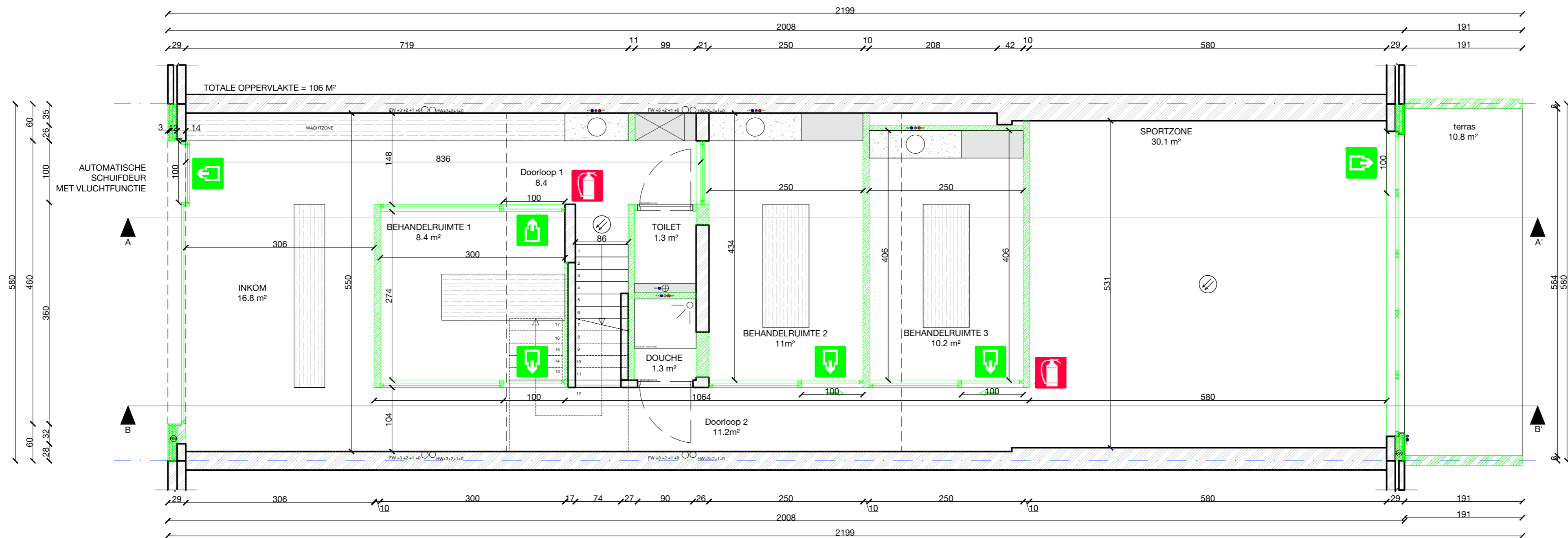
GRONDPLAN GELIJKVLOERS- VERGUNDE SITUATIE (reeds verleend) 1:50
