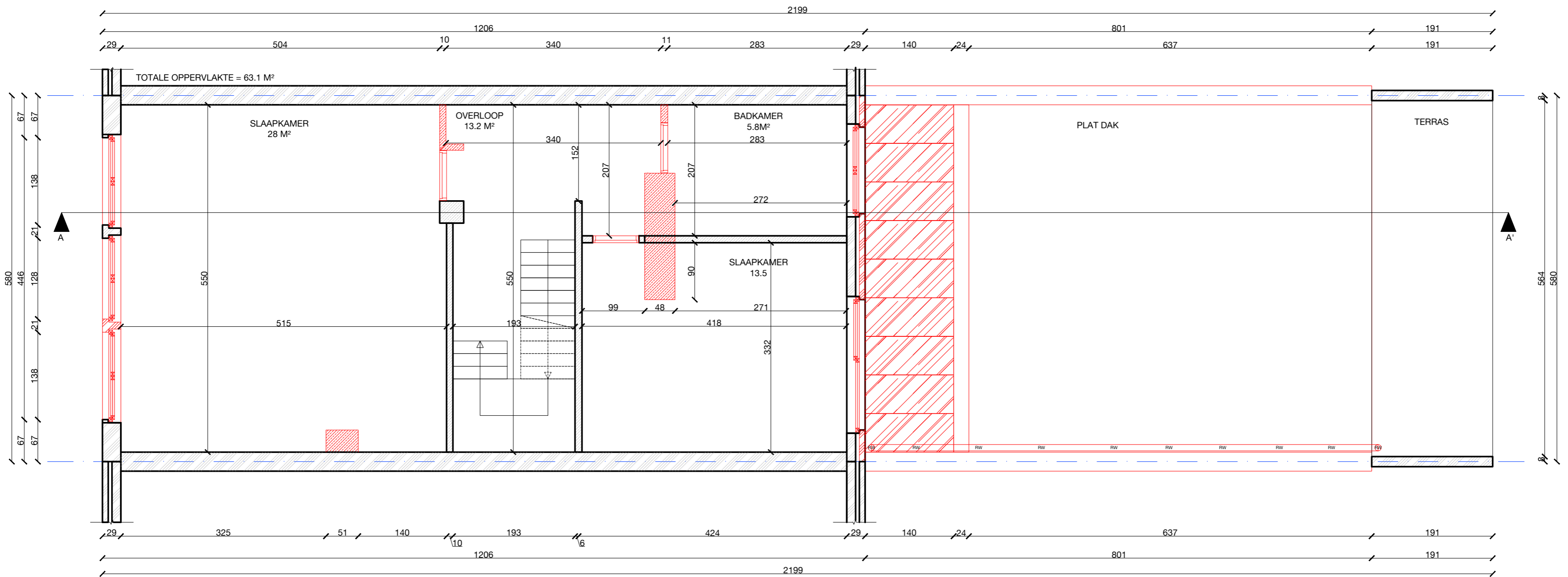
GRONDPLAN VERDIEPING +2- BESTAANDE SITUATIE 1:50
