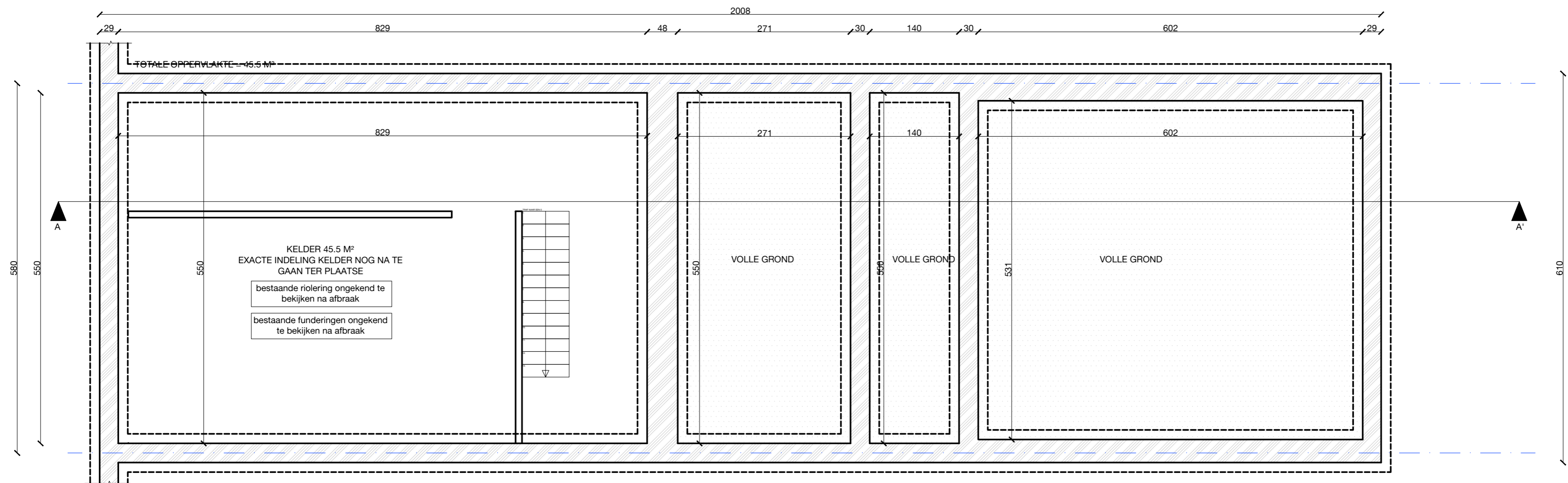
GRONDPLAN KELDER- BESTAANDE SITUATIE 1:50
