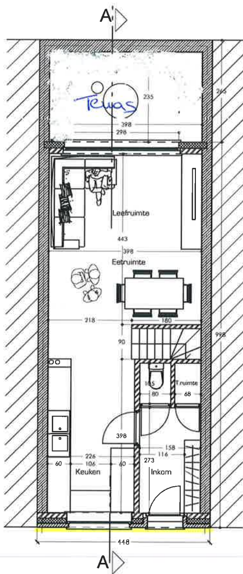
Gelijkvloers +0 nieuw 1/100
