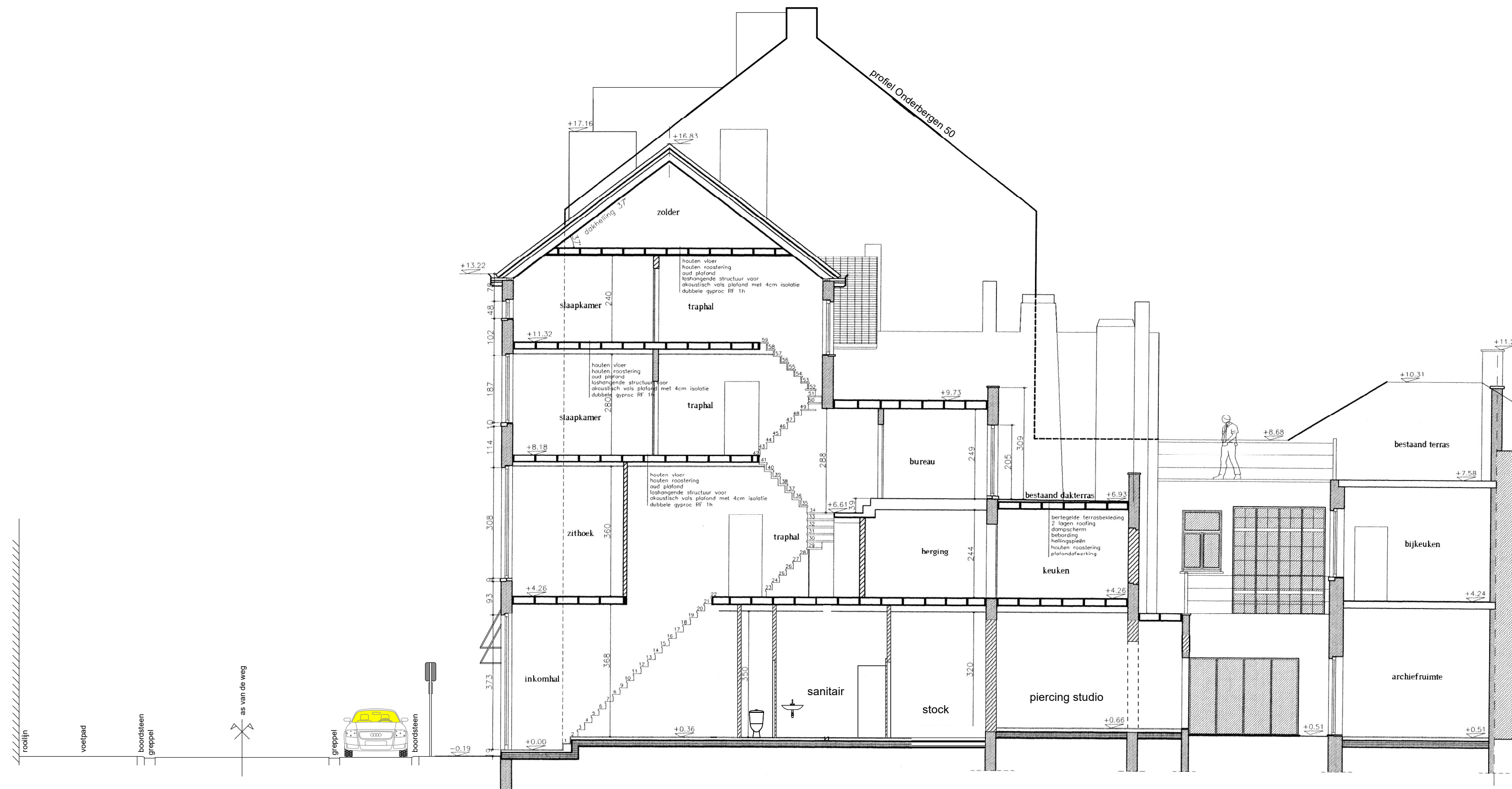
bestaande toestand DOORSNEDE - AA
