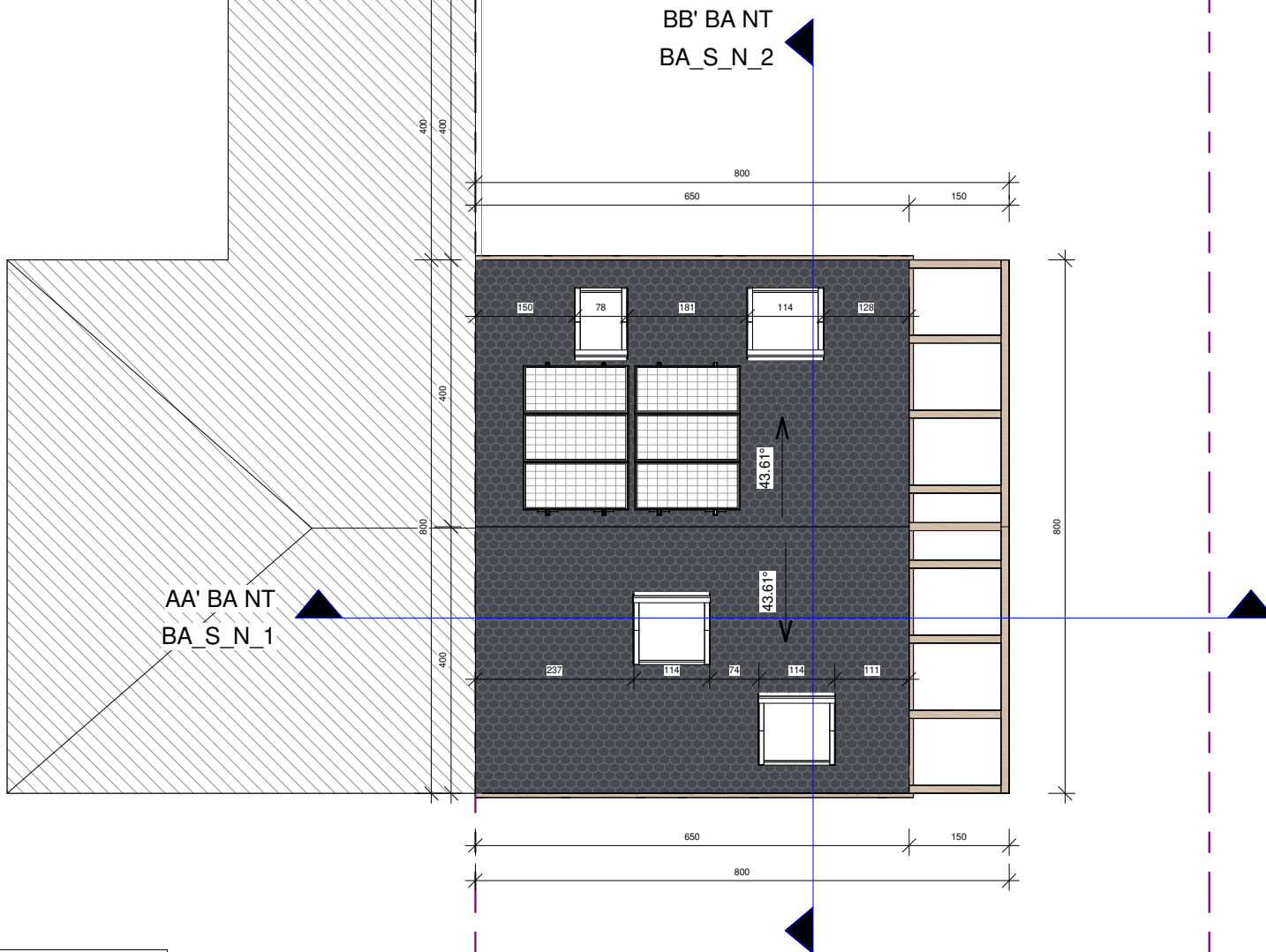
1 1 : 100 50 Dakenplan BA NT
