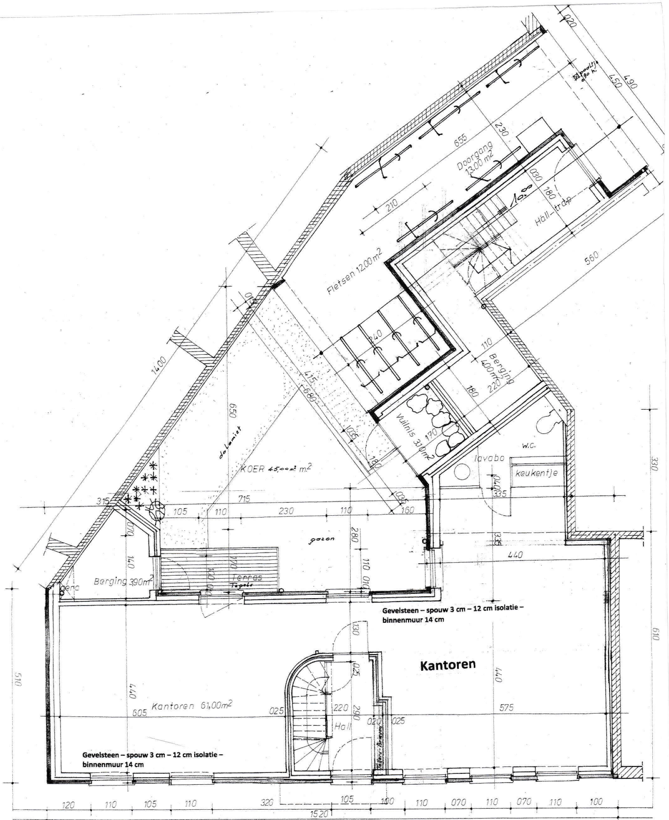
BA_Afbreken 2 gebouwen bouwen eengezinswoning 2 appartementen en kantoren P_N_01_gelijkvloers schaal 1/100 1/200
