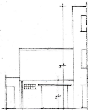
BA_Afbreken 2 gebouwen bouwen eengezinswoning 2 appartementen en kantoren _ G_B_03_voorgevel Borloutstraat schaal 1/100 1/200
