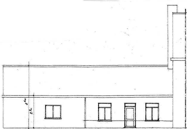
BA_Afbreken 2 gebouwen bouwen eengezinswoning 2 appartementen en kantoren _ G_B_02_voorgevel Loofblommestraat schaal 1/100 1/200
