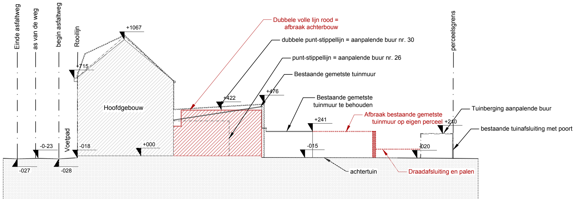
Terreinprofiel - bestand
