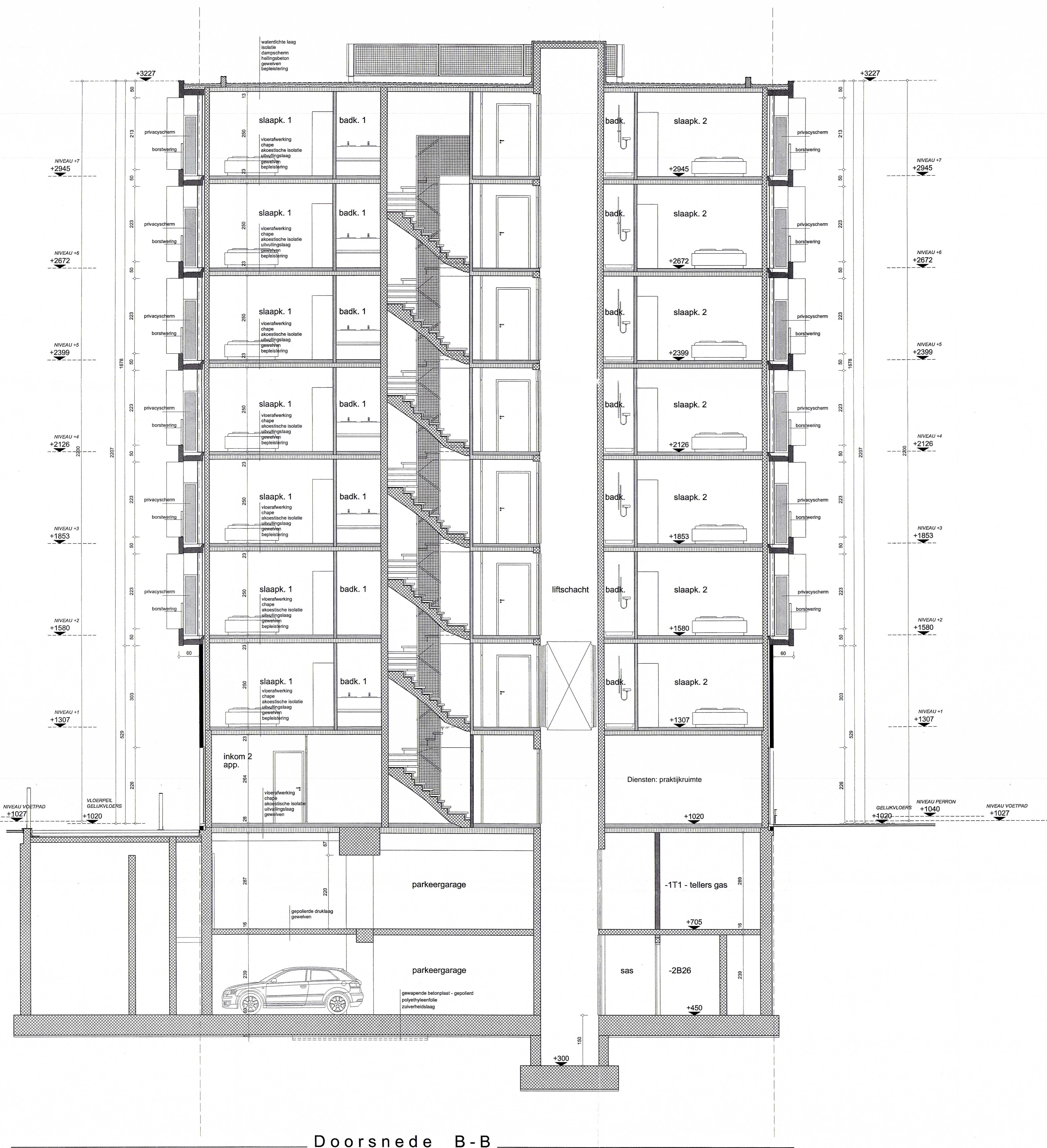
Doorsnede B-B
