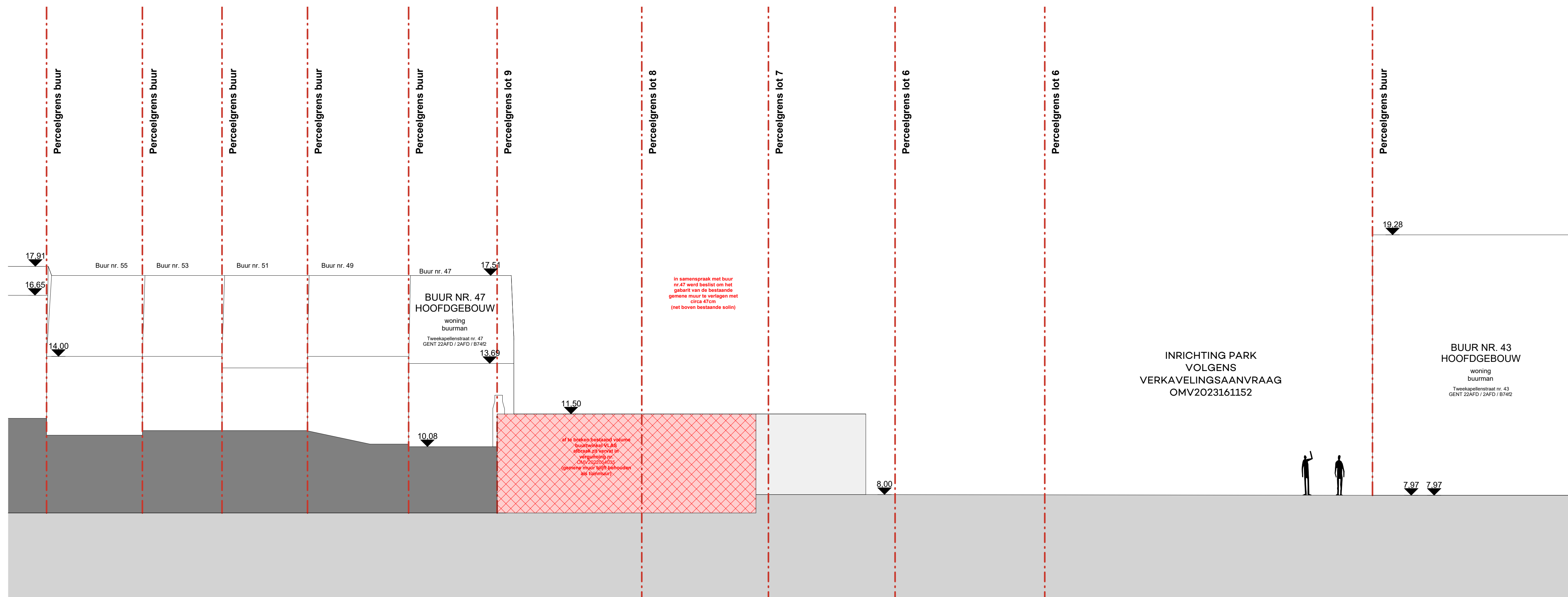
Terreinsnede C-C BT schaal: 1 : 100
