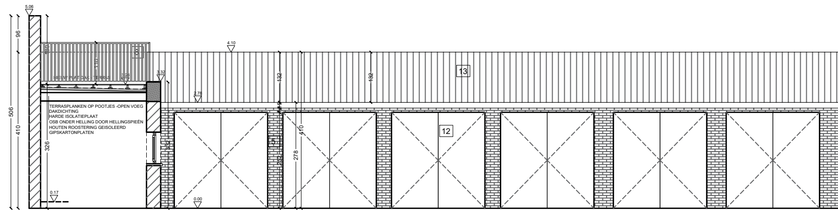
SNEDE A-AA' - GEVEL GARAGES BINNENPLEIN
