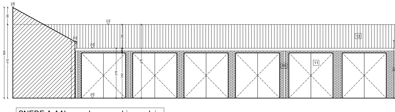
SNEDE A-AA' - gevel garages binnenplein
