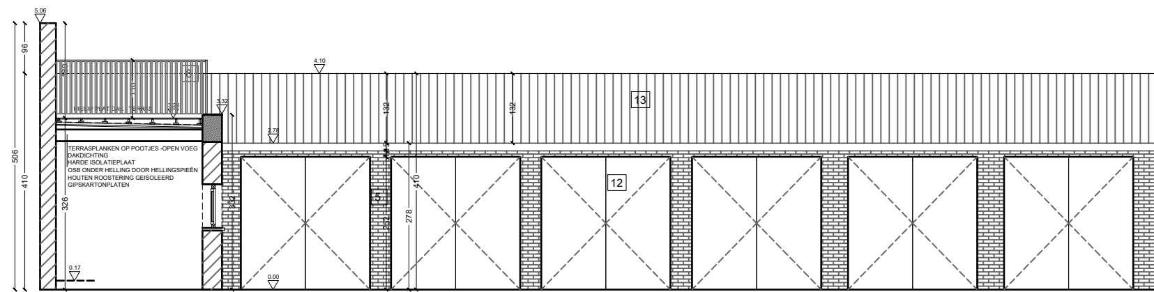
SNEDE A-AA' - GEVEL GARAGES BINNENPLEIN
