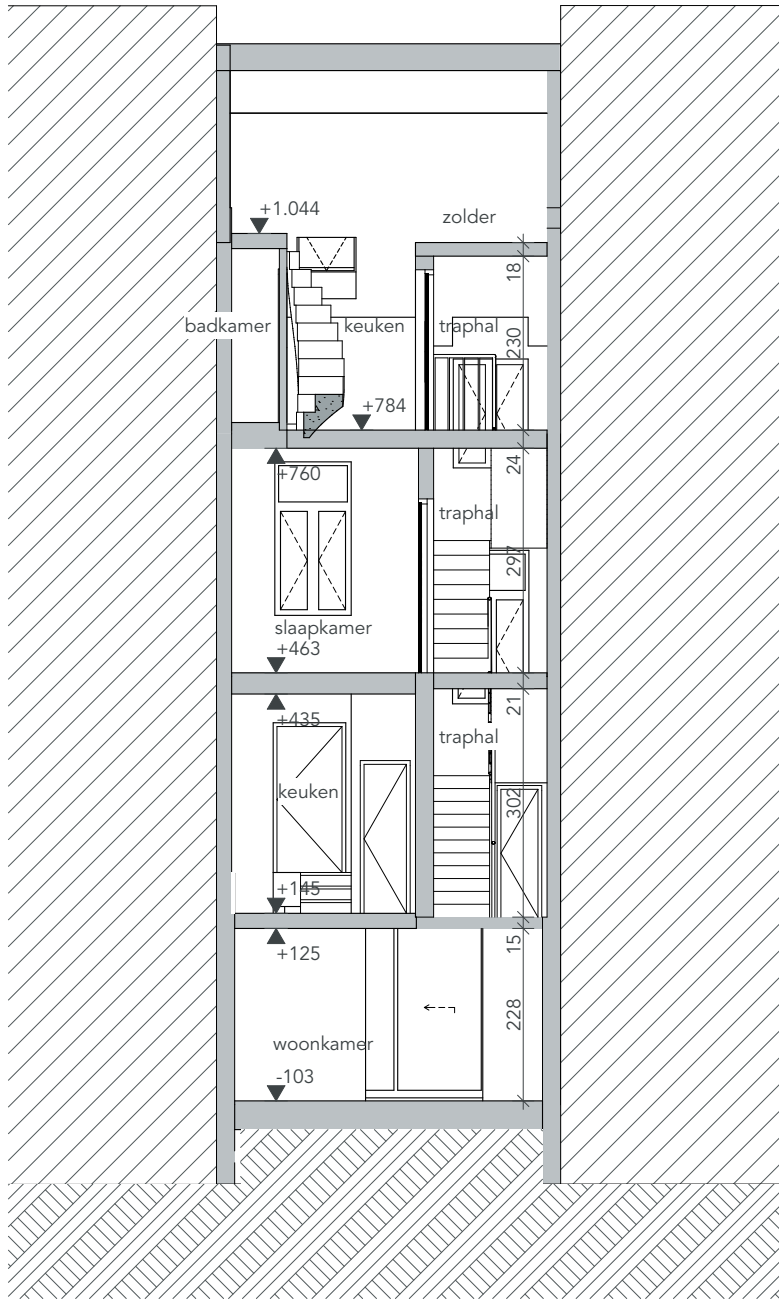
0 1 2 3 4 BT Doorsnede A-A
